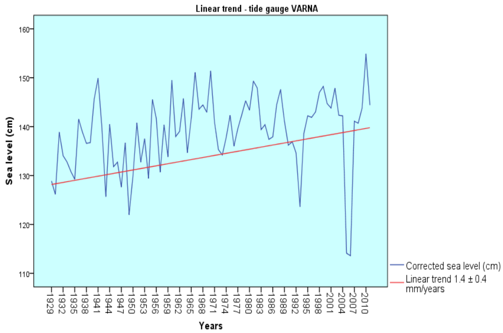
Изменение на морското ниво в мареографна станция Варна за периода 1928 – 2011 година
